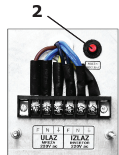
Izgled priključne kutije sa rasporedom kleva
